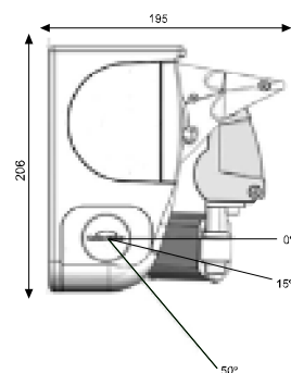
Inclinación máxima con semicofre
