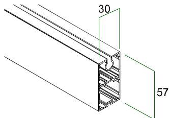
Kit perfiles guía Zip
