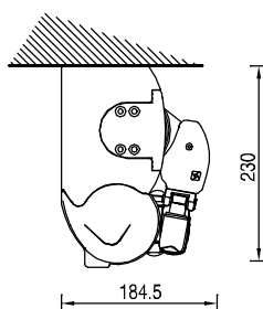
Montaje a techo
