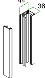
Kit perfiles guía Zip
