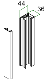
Kit perfiles guía Zip
