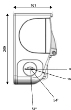
Inclinación máxima
