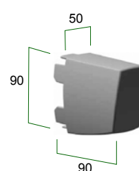
Terminal perfil 90 x 50 (pecho palomo)
