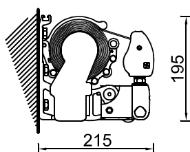
Montaje a pared
