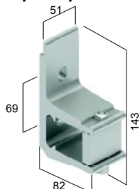
Soporte pared
