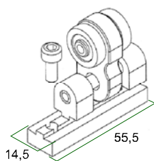
Polea corredera
