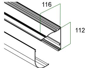
Perfiles cofre 110
