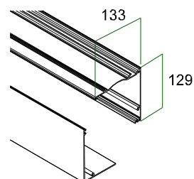
Perfiles cofre 130
