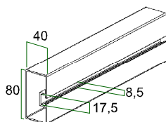
Perfil 80x40 con ranura
