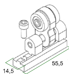
Polea corredera
