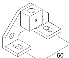
Jgo. pies para guiado
