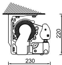
Montaje a techo
