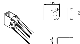
Soporte pared motor
