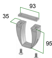
Brida unión en u
