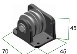
Polea esquina
