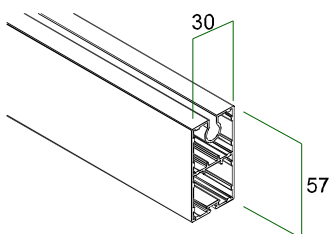
Perfil de carga Tambre
