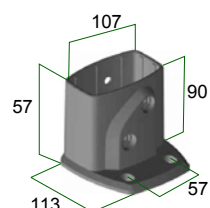
Soporte suelo 90 x 50
