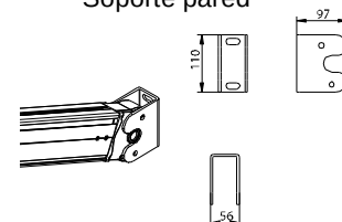
Soporte pared
