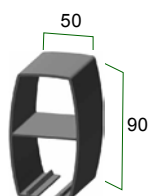
Perfil guía 90 x 50
