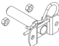
Pivote extraíble
