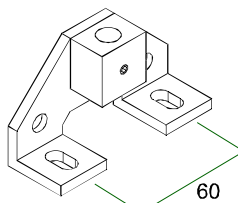
Jgo. pies para guiado
