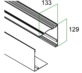
Perfiles cofre 130
