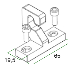
Gancho final
