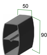
Perfil 90 x 50
