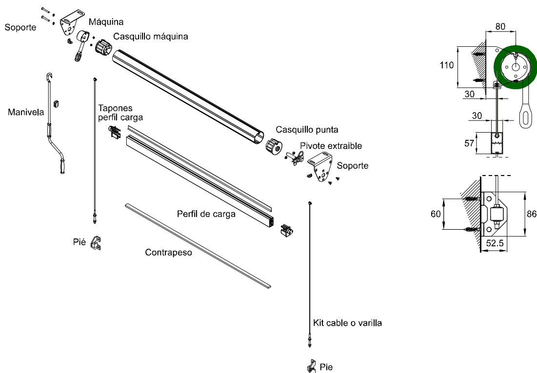
Jgo. de soportes Tambre
